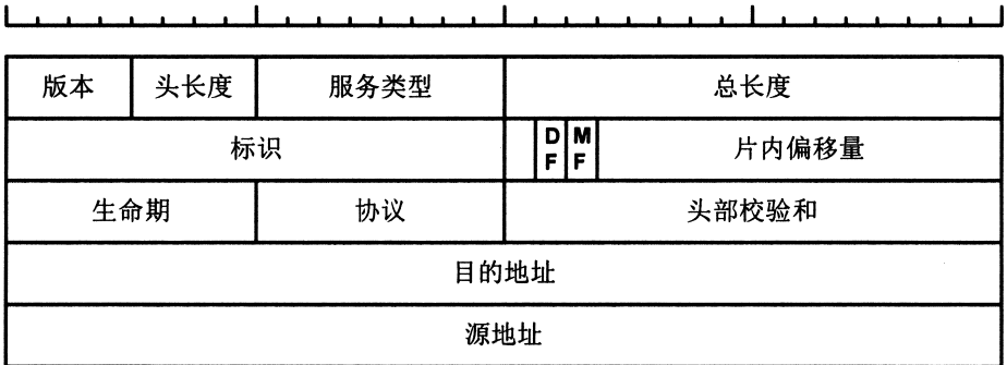
题 47 图 1 IP 头部格式
